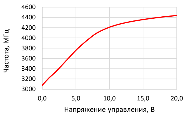
Рисунок 1 – диапазон перестройки
