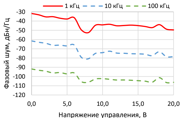
Рисунок 6 – фазовый шум
