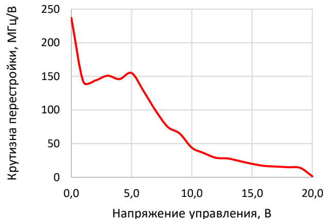
Рисунок 2 – крутизна перестройки
