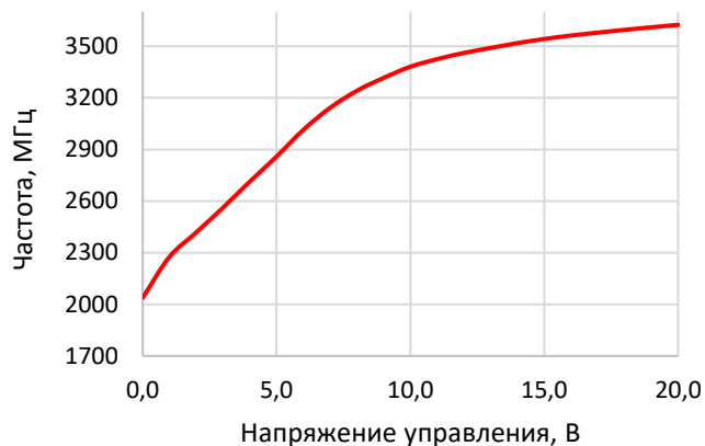
Рисунок 1 – диапазон перестройки
