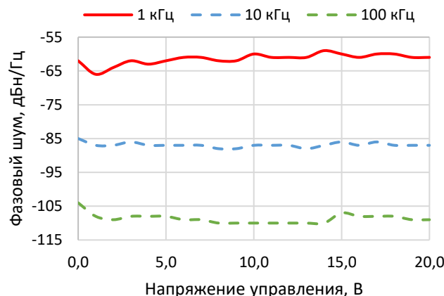
Рисунок 6 – фазовый шум
