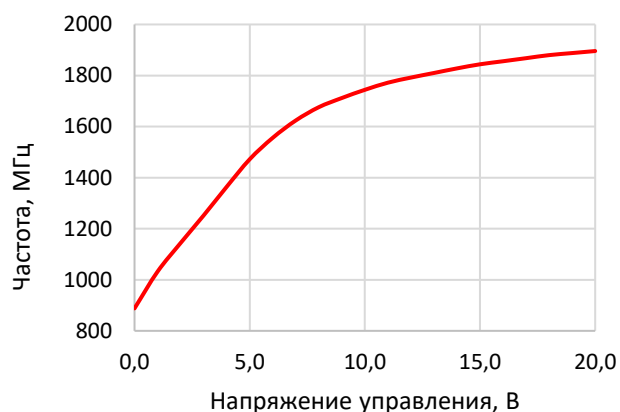
Рисунок 1 – диапазон перестройки
