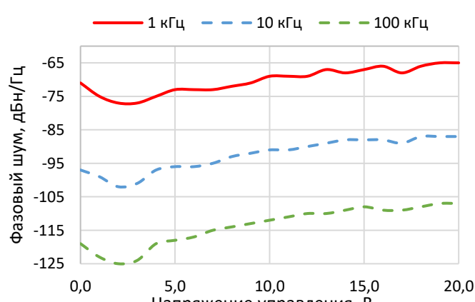
Рисунок 6 – фазовый шум
