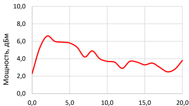
Рисунок 4 – выходная мощность
