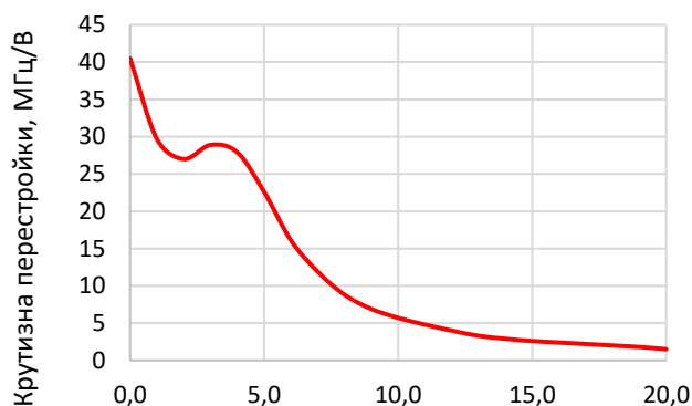
Рисунок 2 – крутизна перестройки
