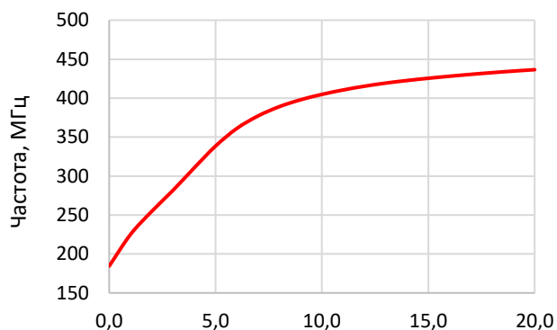
Рисунок 1 – диапазон перестройки
