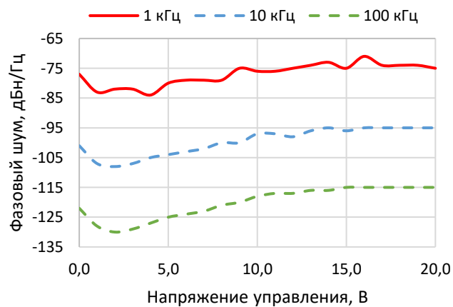
Рисунок 6 – фазовый шум
