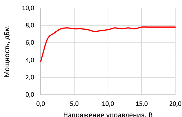
Рисунок 4 – выходная мощность
