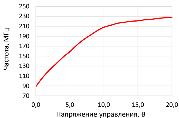
Рисунок 1 – диапазон перестройки
