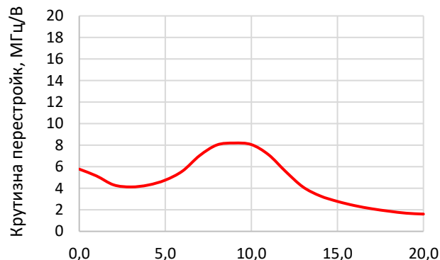
Рисунок 2 – крутизна перестройки
