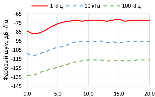
Рисунок 6 – фазовый шум
