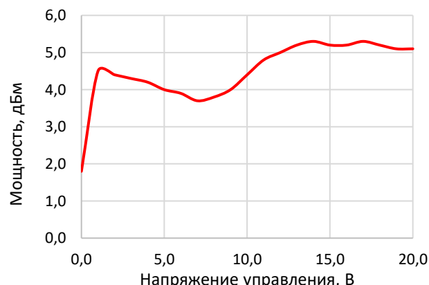
Рисунок 4 – выходная мощность
