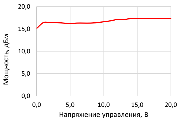
Рисунок 3 – выходная мощность
